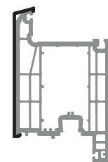
3318 385 gr/m Al cover cap door sash
